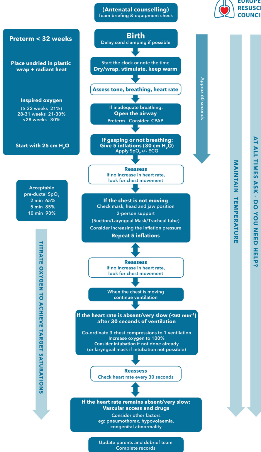
Fig. 5 – NLS algorithm.
